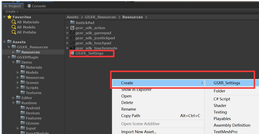
图 23 生成 GSXR_Settings
