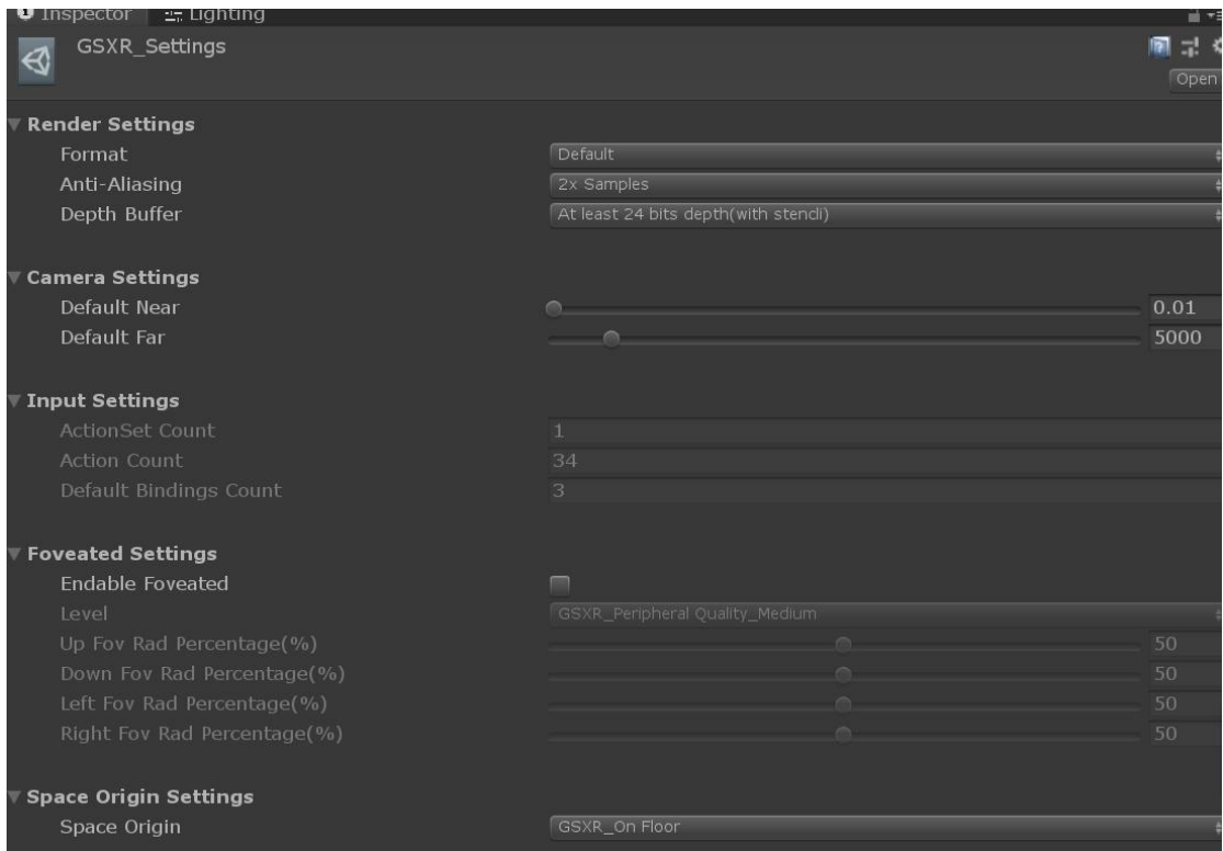
图 25 修改 GSXR_Settings
