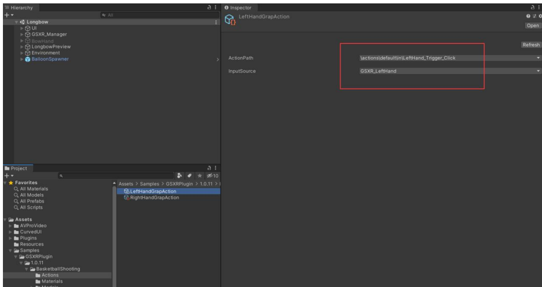
图 39 设置 ActionData
