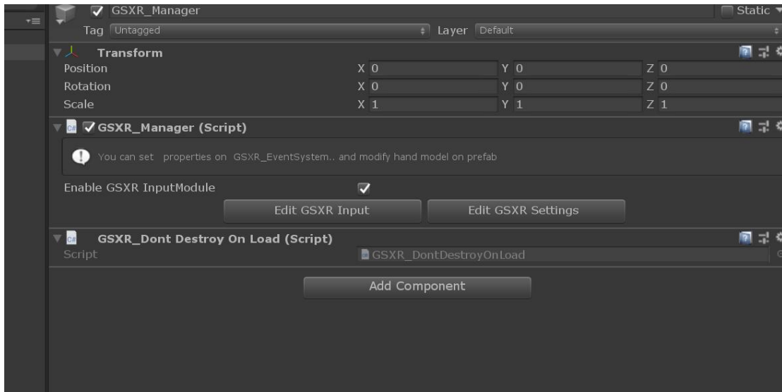
图 27 DontDestroyOnLoad 绑定
