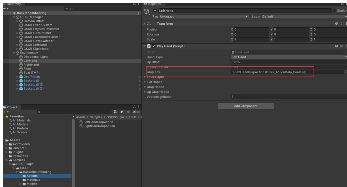
图 40 绑定 ActionData
