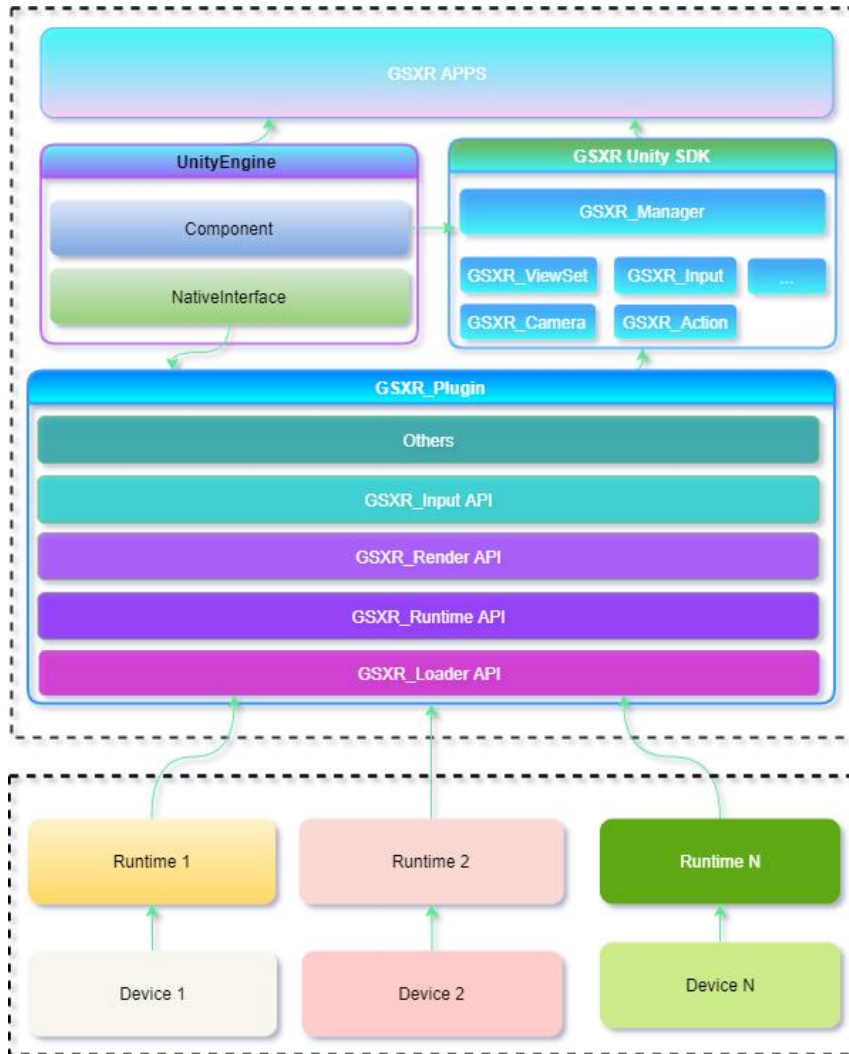
图 1 SDK 架构图
