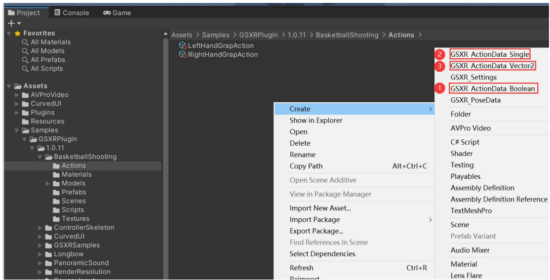
图 38 生成 ActionData
