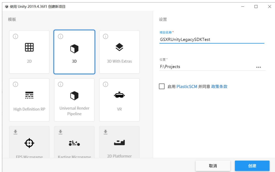
图 8 新建工程
